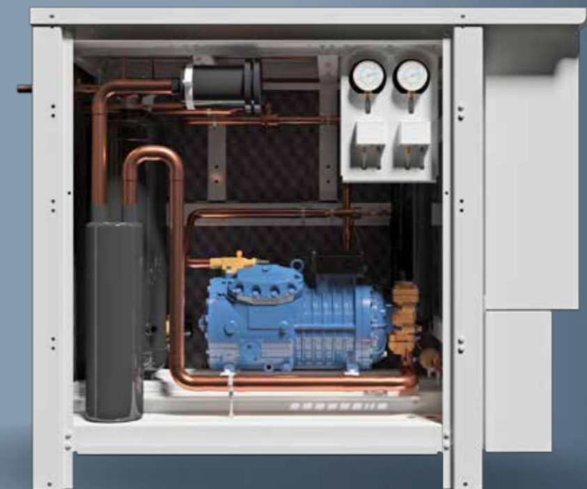
ЦХМ на базе поршневых компрессоров
